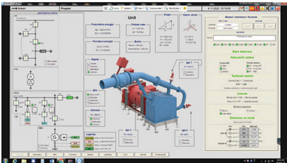
Slika 7: SCADA sistem MHE Krkori
