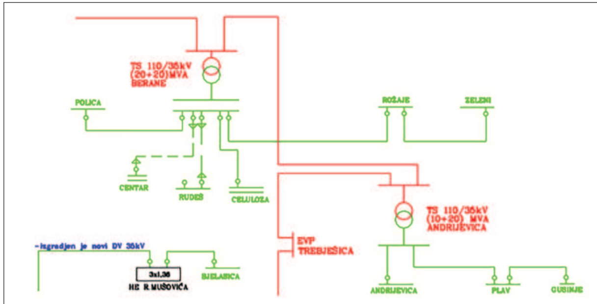
Slika 10: Sistem napajanja
