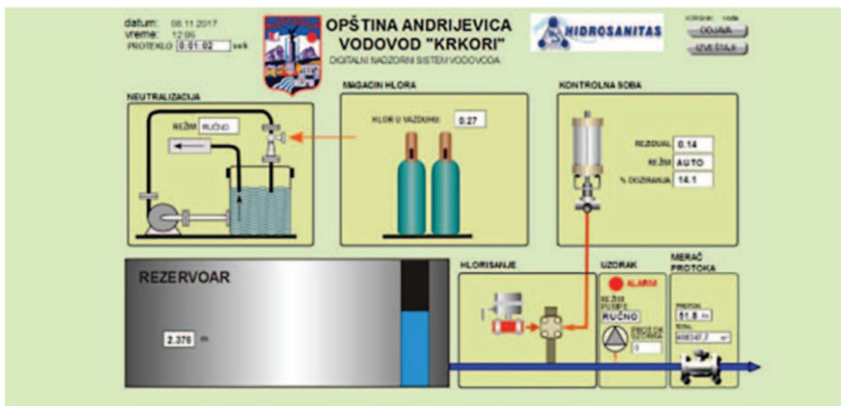
Slika 6: Prikaz hlorisanja vode SKADA sistema
