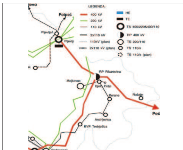
Slika 9: Energetska shema napajanje Andrijevice
